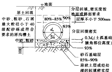
图 1 沟槽各部位回填土要求
